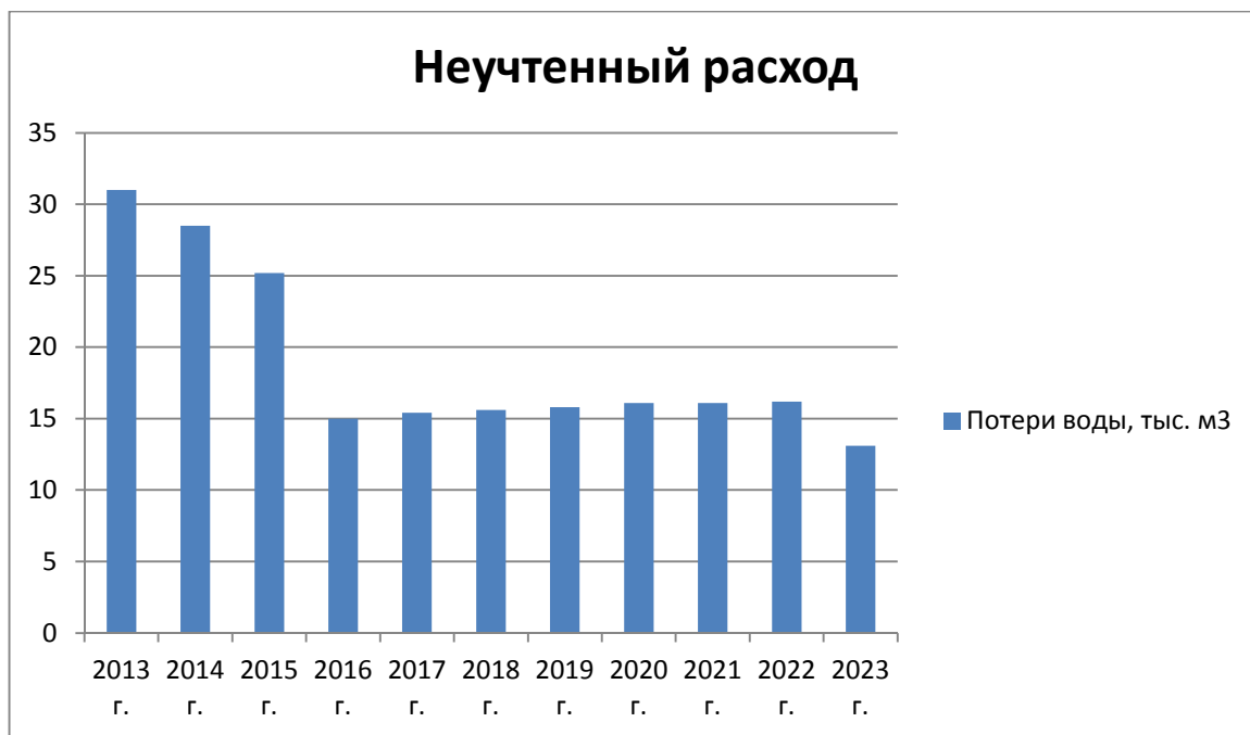
Рис.4. Утечки и неучтенный расход воды.
